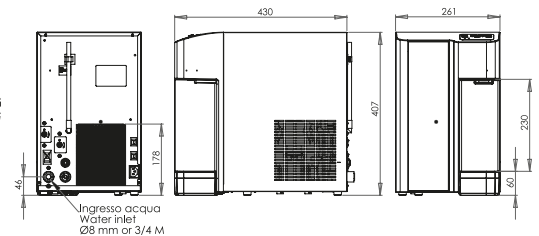
Versioni CHWG Version CHWG
